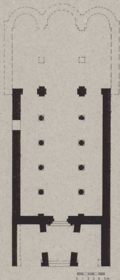
Fig. 12 Ipotesi ricostruttiva finale disegnata in considerazione delle tracce superficiali rinvenute nel corso dei sopralluoghi
