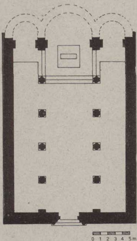
Fig. 6 Prima ipotesi di parte absidale disegnata in rapporto allo sviluppo modulare dell'impianto
