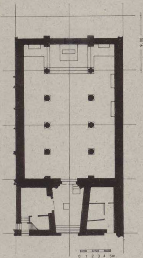
Fig. 5 La "maglia" ripartita in otto moduli sovrapposti alla pianta della chiesa
