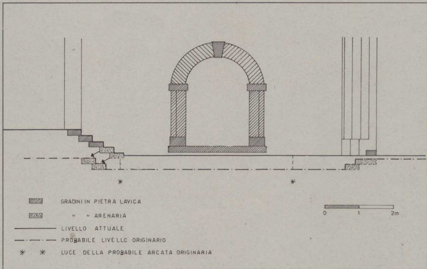
Fig. 13 Sezione del vano centrale del narthex
