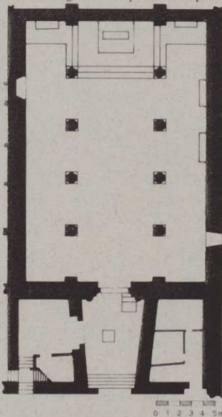
Fig. 2 Rilievo in pianta della chiesa nello stato e nelle dimensioni odierne
